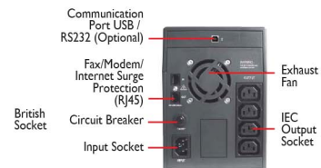
BP1K0E - BP2K2E (Rear Panel)
