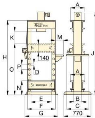
XLP 25 ton
