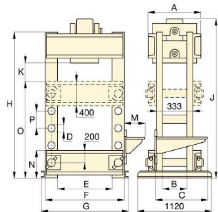
VLP 200 ton
