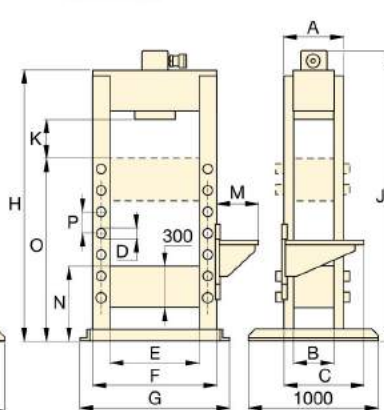
VLP 100 ton
