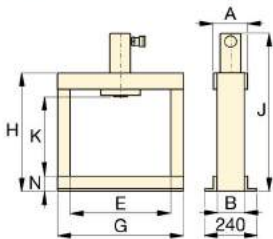
VLP 10 ton
