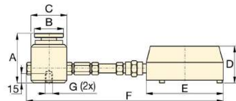
LH-Series
