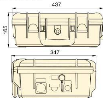
ETWCB-control box
