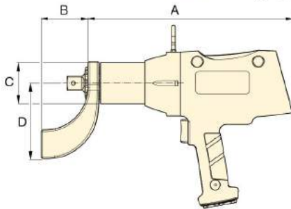
ETW-torque wrench
