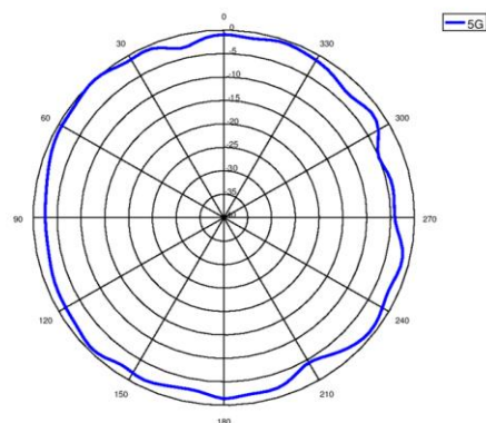
5G-2 (PHI=0)
