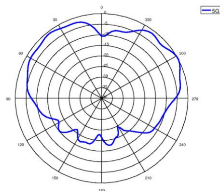
5G-2 (PHI=90)
