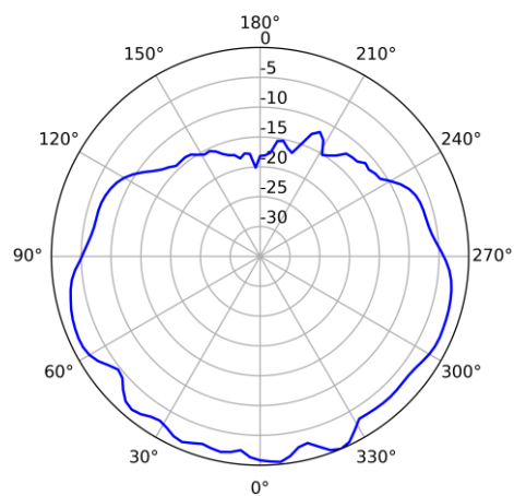
5GHz (Vertical)
