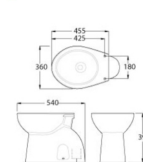
WC1037 Spin WC
