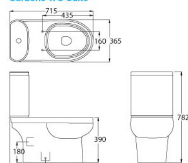
WC1040 Carbene WC Suite
